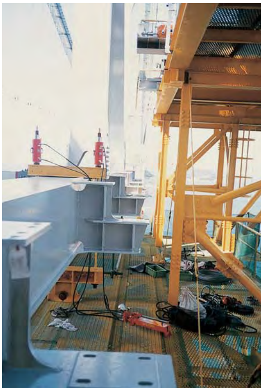
中空ジャッキでハンガーの引込中 (EC100H15&TWAD-4を使用)
