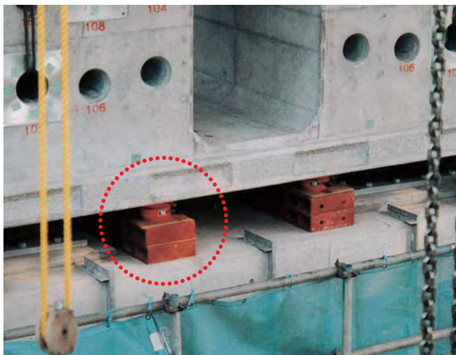
橋桁のシュー取替え用 (JFN200S3&TWA-1.3PGを使用)
