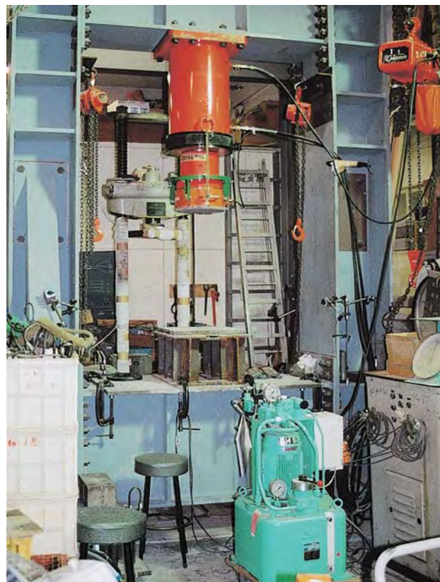
大学研究室での耐荷挙動特性の解明研究用 (5000kN×300st油圧ジャッキ&GH5-Pを使用)
