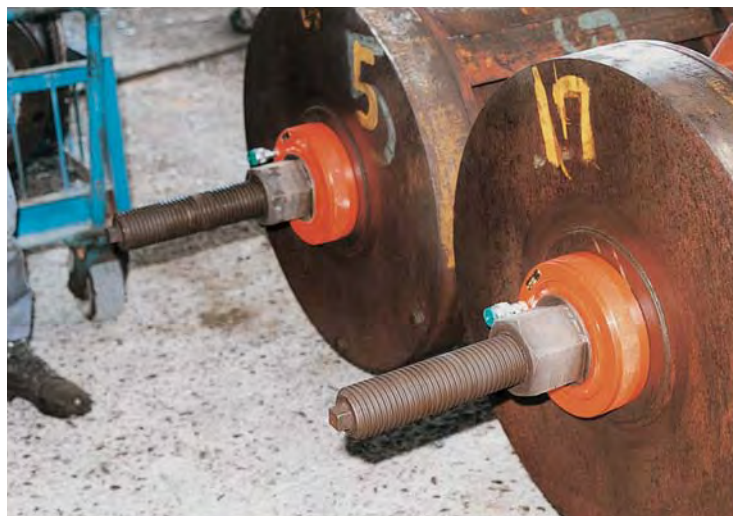
緊張用油圧ワッシャを型枠にセット中
