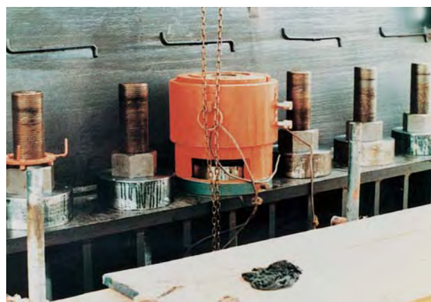
橋脚のボルト締付け用 (500kN×20stボルトテンシヨナを使用)
