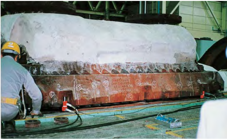
タービンのジャッキアップ用 (200kN×700stパワージャッキ&同調ポンプを使用)
